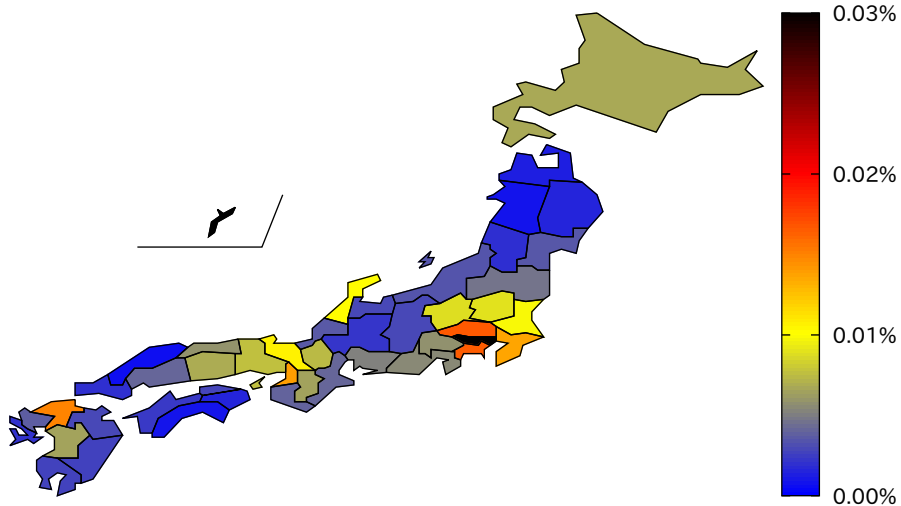
都道府県人口当たりの新規感染者数 (2021/8/4)
