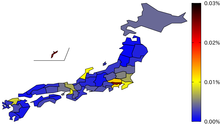
都道府県人口当たりの新規感染者数 (2021/7/28)
