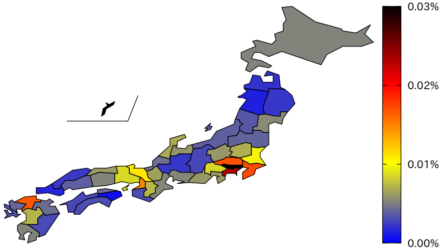
都道府県人口当たりの新規感染者数 (2021/8/6)
