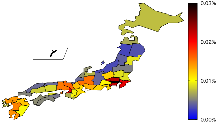
都道府県人口当たりの新規感染者数 (2021/8/17)
