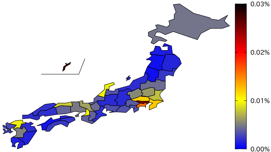
都道府県人口当たりの新規感染者数 (2021/7/30)
