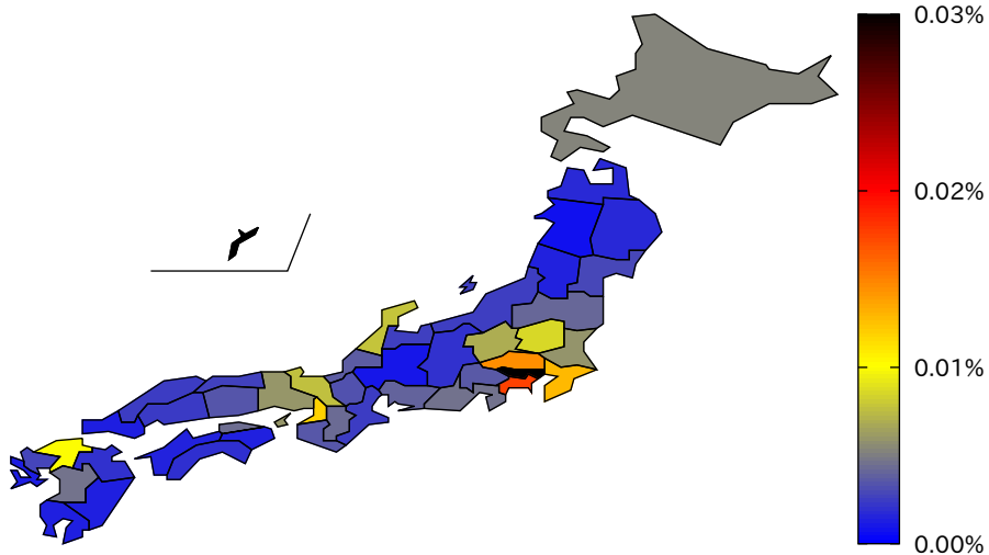
都道府県人口当たりの新規感染者数 (2021/7/31)
