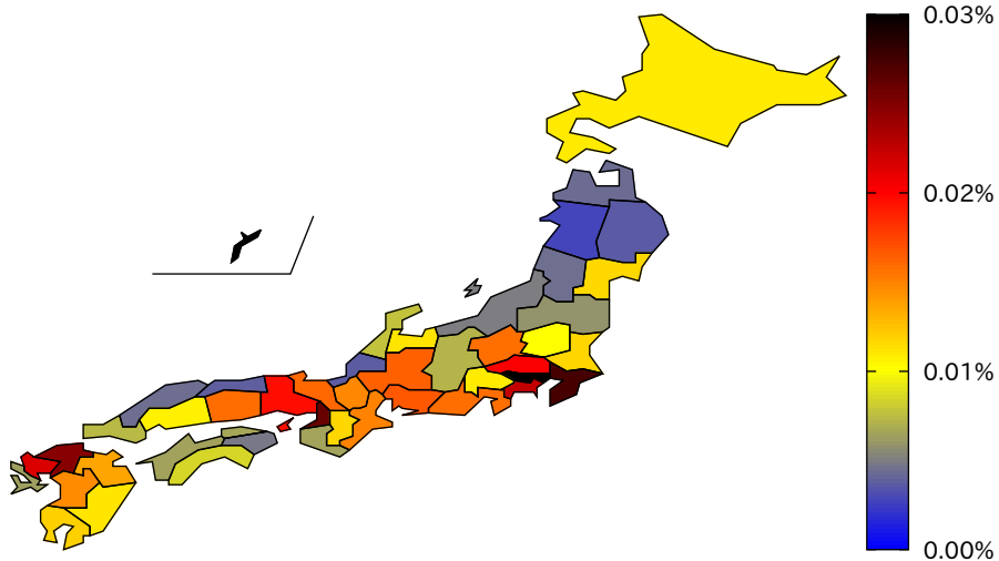
都道府県人口当たりの新規感染者数 (2021/8/18)
