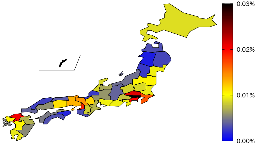
都道府県人口当たりの新規感染者数 (2021/8/12)
