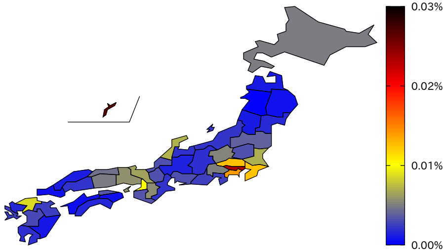
都道府県人口当たりの新規感染者数 (2021/8/1)
