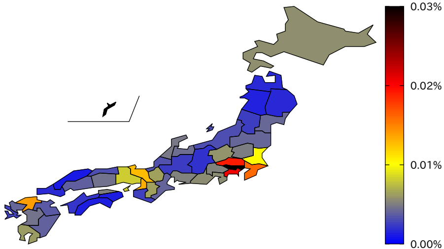
都道府県人口当たりの新規感染者数 (2021/8/8)
