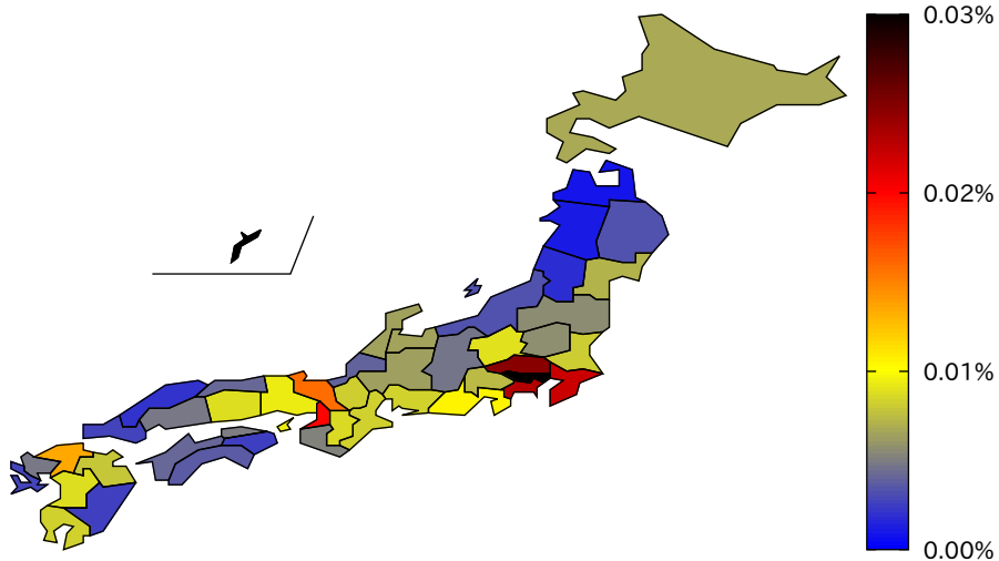
都道府県人口当たりの新規感染者数 (2021/8/15)
