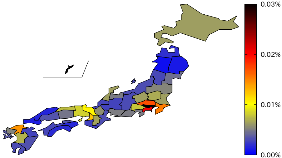
都道府県人口当たりの新規感染者数 (2021/8/5)
