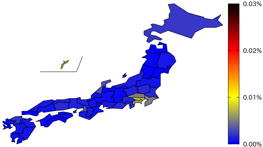
都道府県人口当たりの新規感染者数 (2021/7/24)
