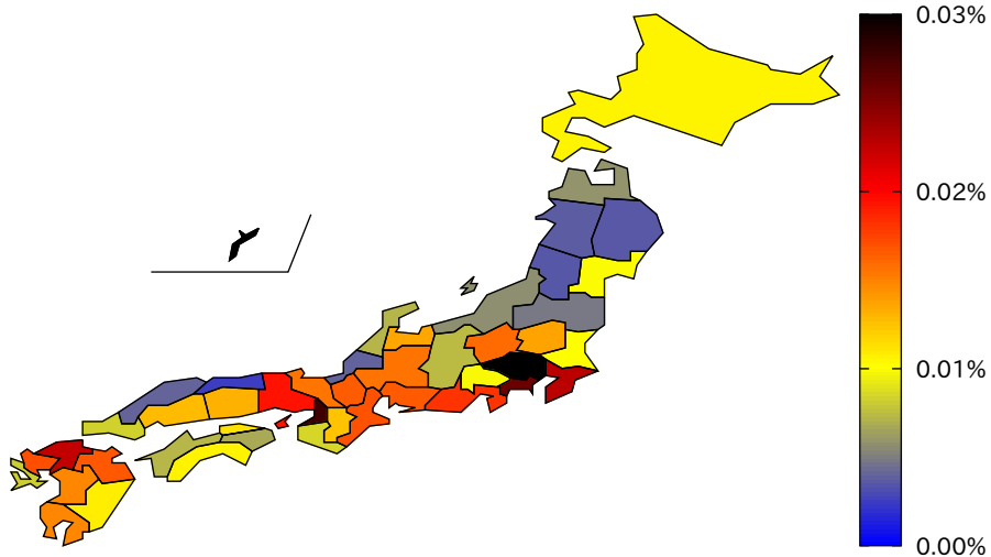
都道府県人口当たりの新規感染者数 (2021/8/19)
