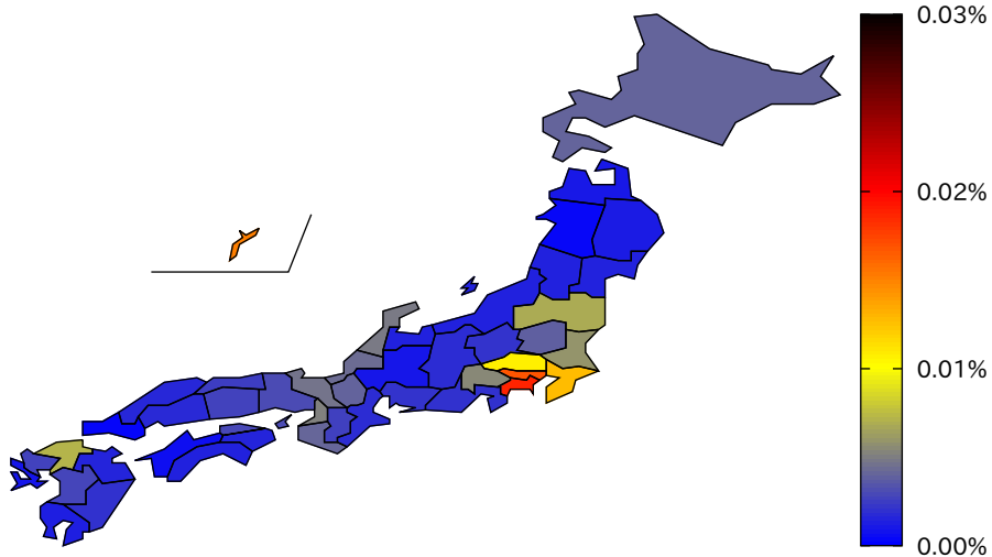
都道府県人口当たりの新規感染者数 (2021/8/2)
