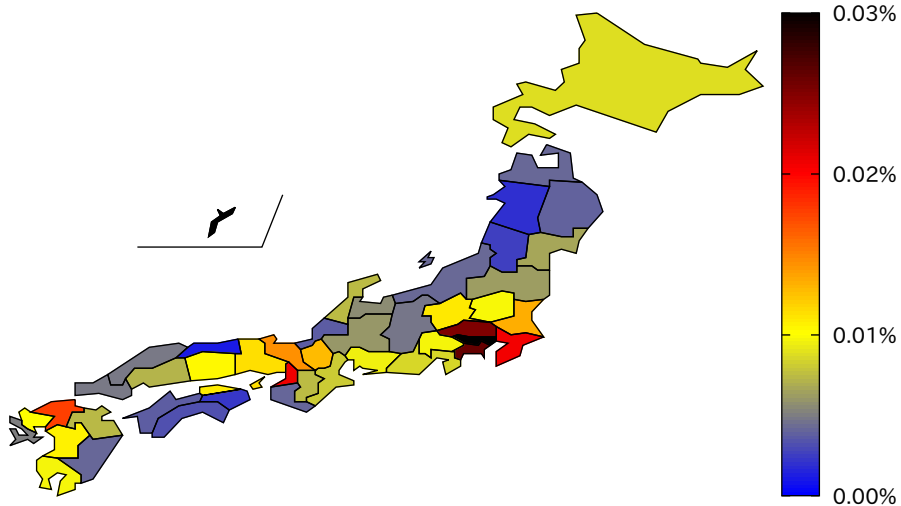
都道府県人口当たりの新規感染者数 (2021/8/14)
