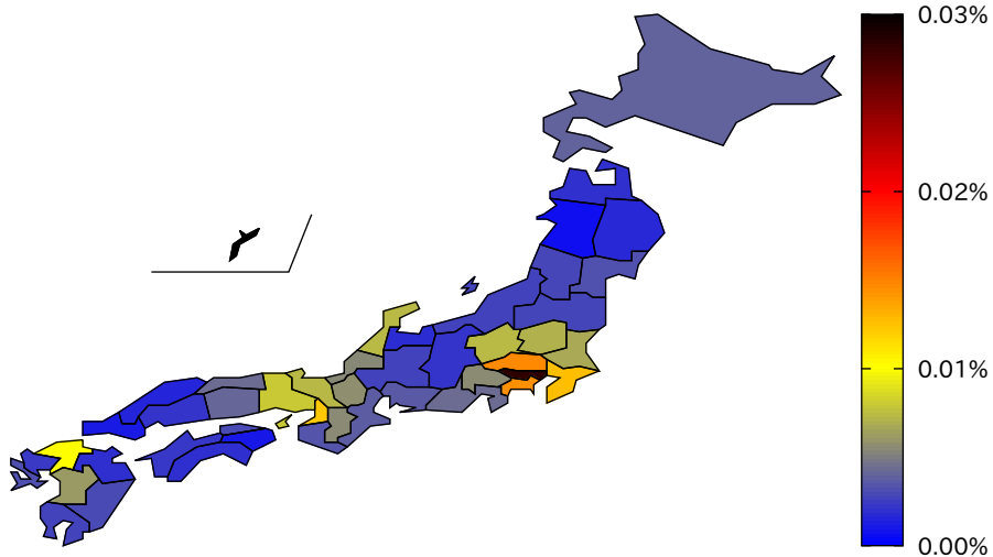
都道府県人口当たりの新規感染者数 (2021/8/3)
