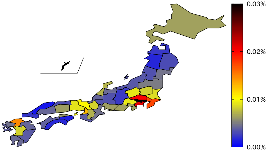
都道府県人口当たりの新規感染者数 (2021/8/7)
