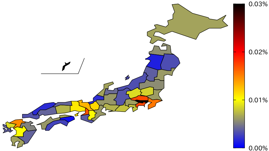
都道府県人口当たりの新規感染者数 (2021/8/11)
