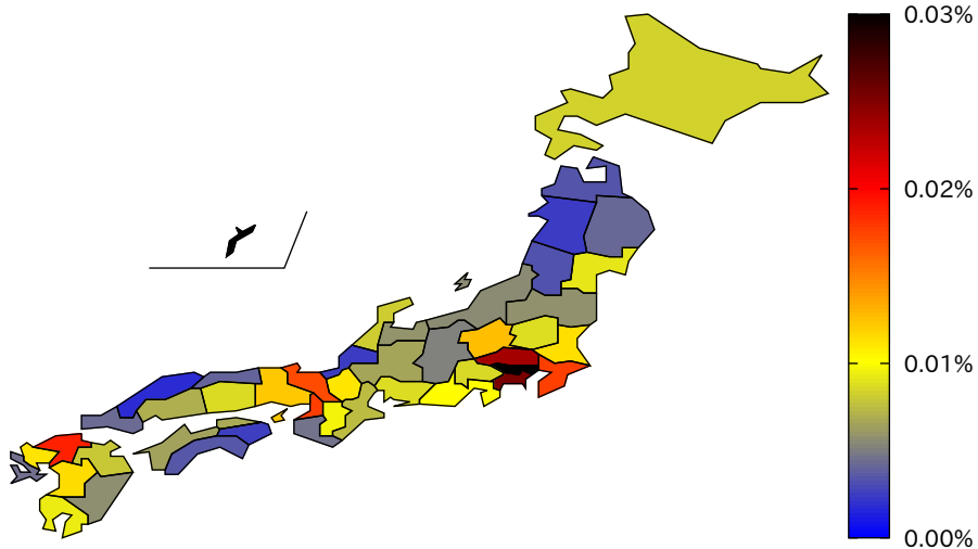
都道府県人口当たりの新規感染者数 (2021/8/13)
