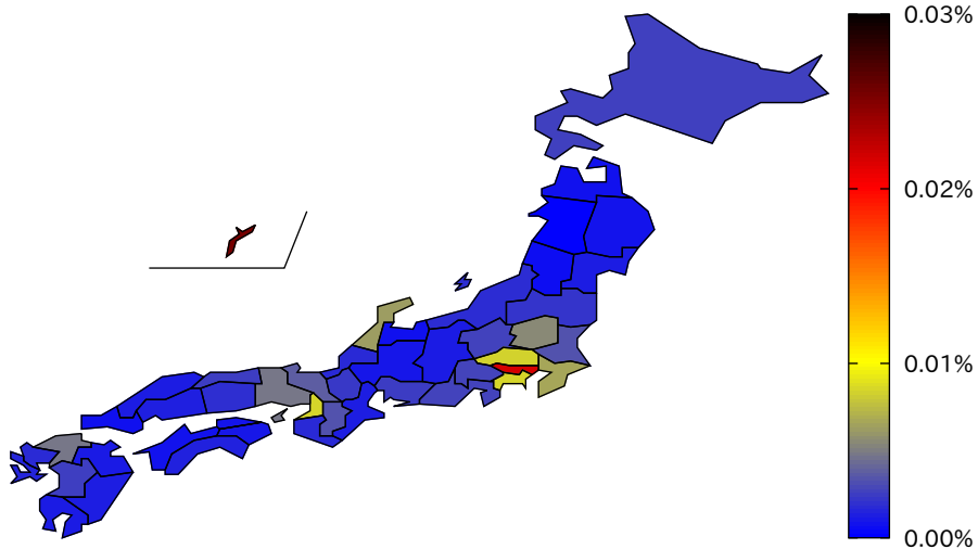
都道府県人口当たりの新規感染者数 (2021/7/27)
