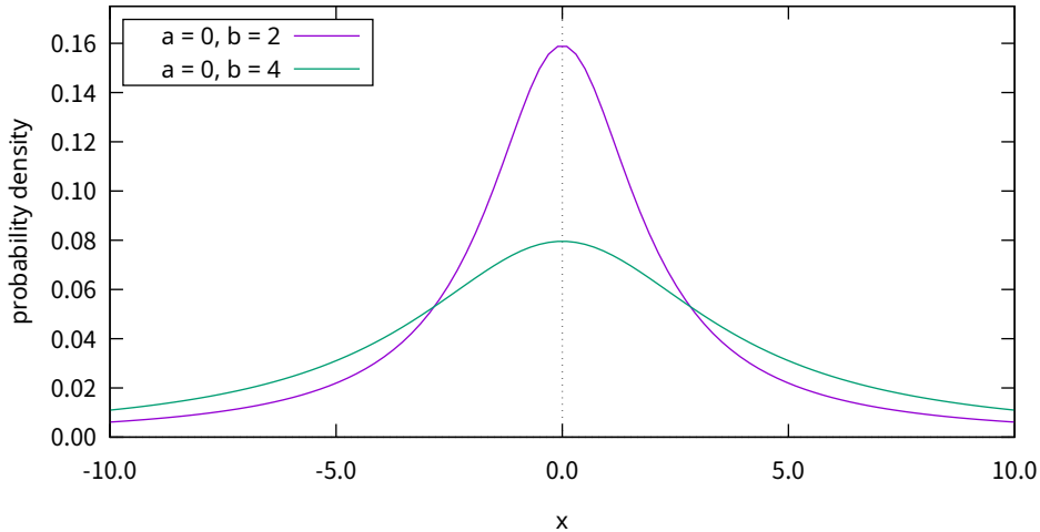
Cauchy PDF
