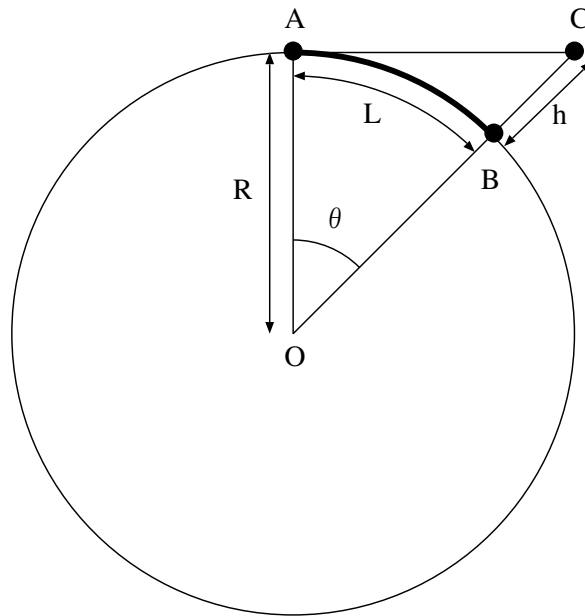
図 1: 地球の図
