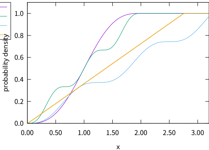
sine CDF
